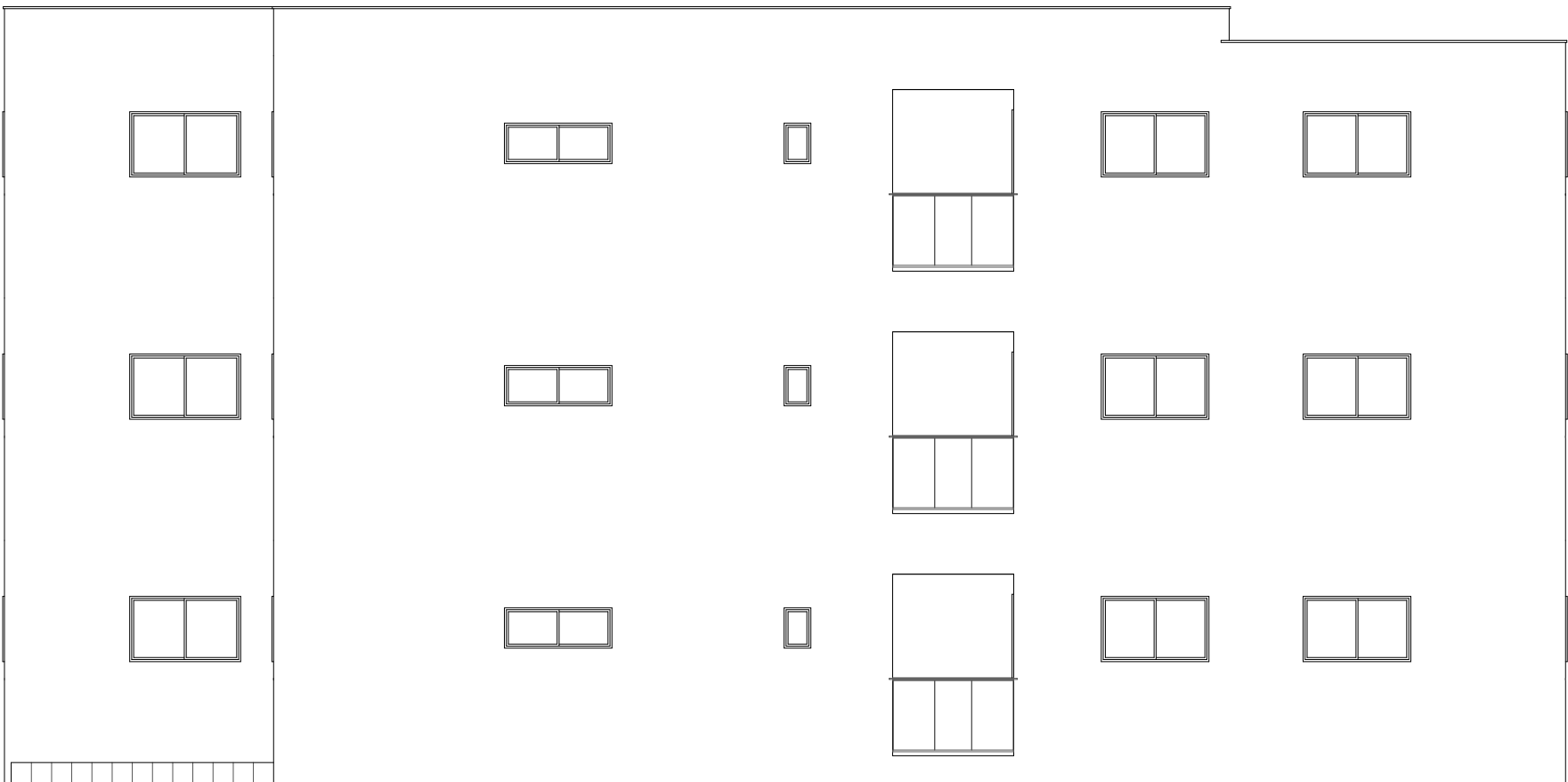
東側立面图 S:1/100
